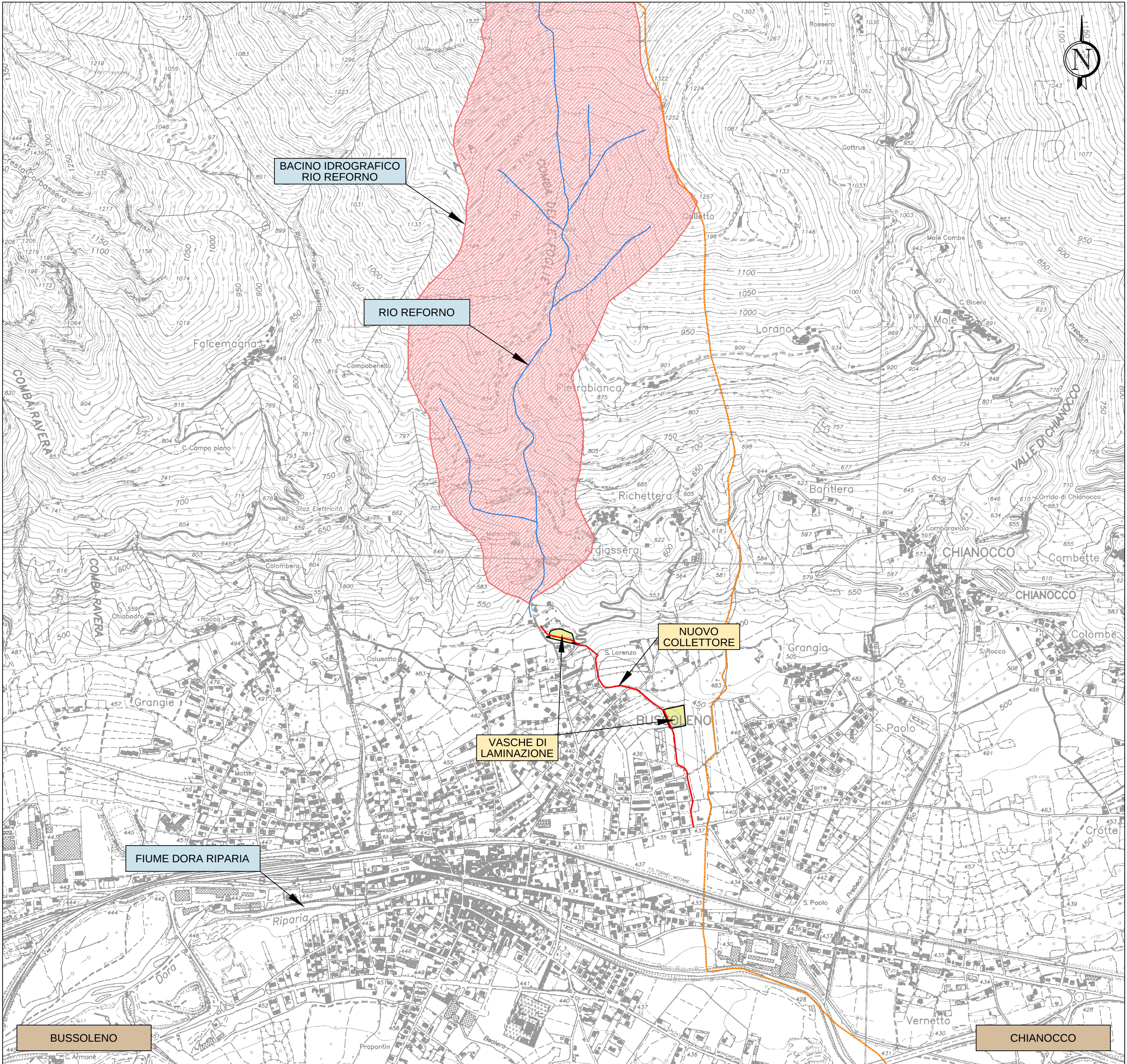
COROGRAFIA Base carta: CARTA TECNICA REGIONALE 1:10.000 Scala 1 : 10.000 0 200 400 600 800 1000 m
