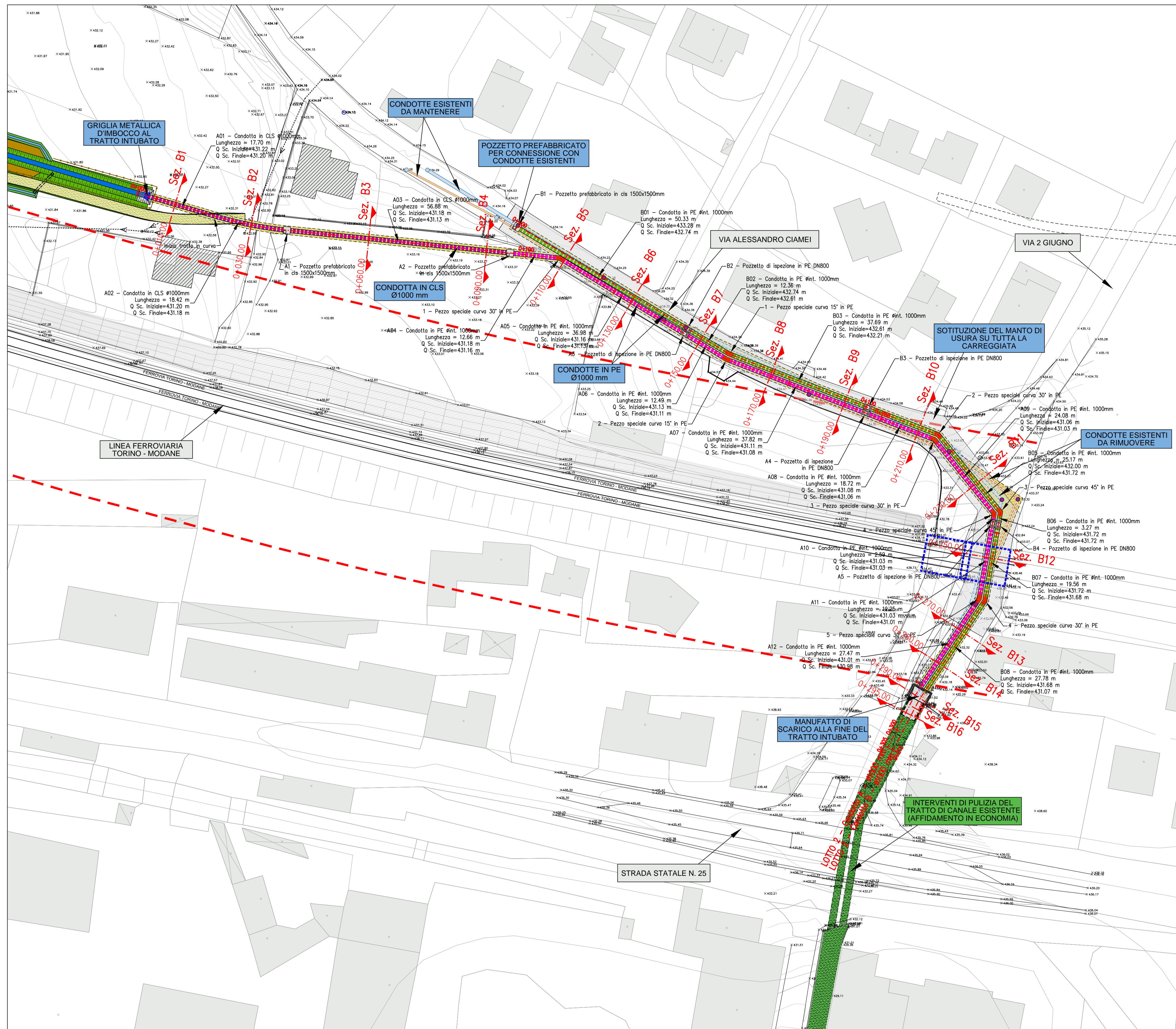
TRATTO INTUBATO - PLANIMETRIA DI PROGETTO Base carta: CARTA TECNICA REGIONALE 1:10.000
